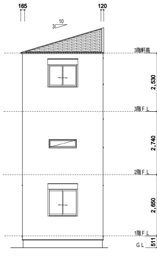
西側 立面図
