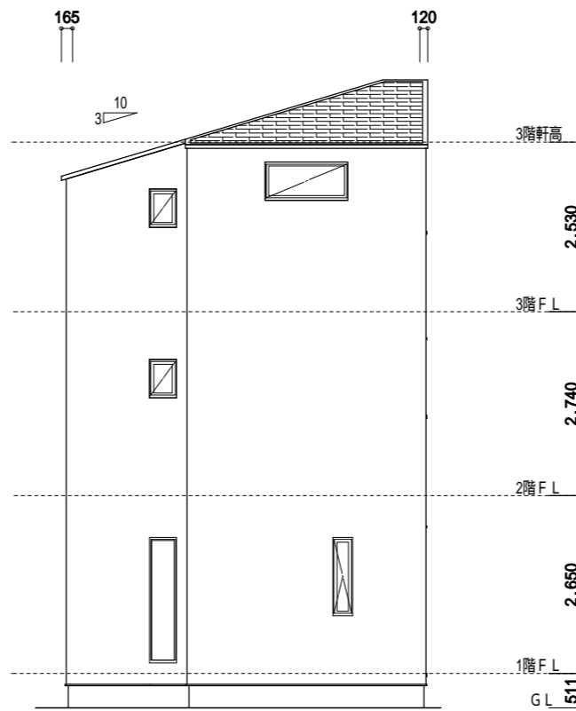
西側立面図
