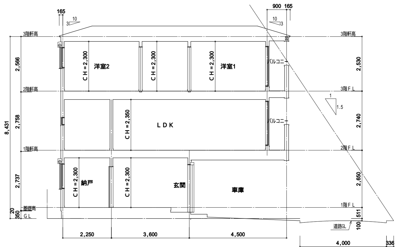
2面 断面図
