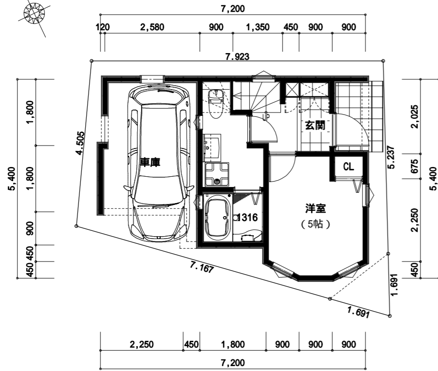
1階 平面図
