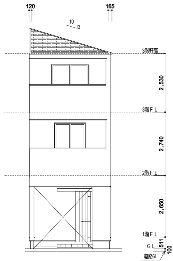
東側 立面図
