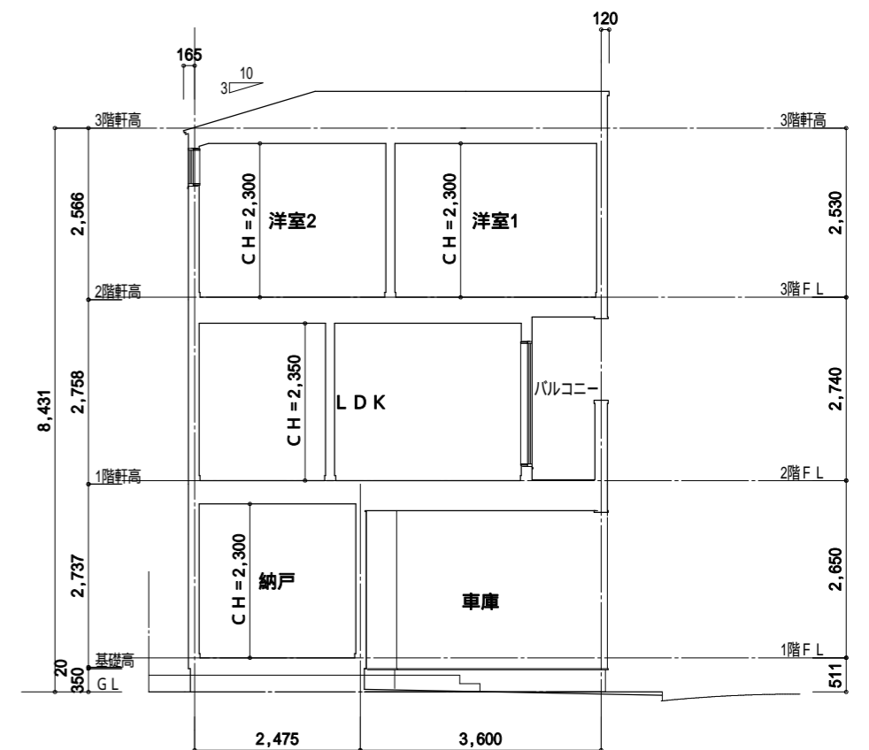
2面断面図
