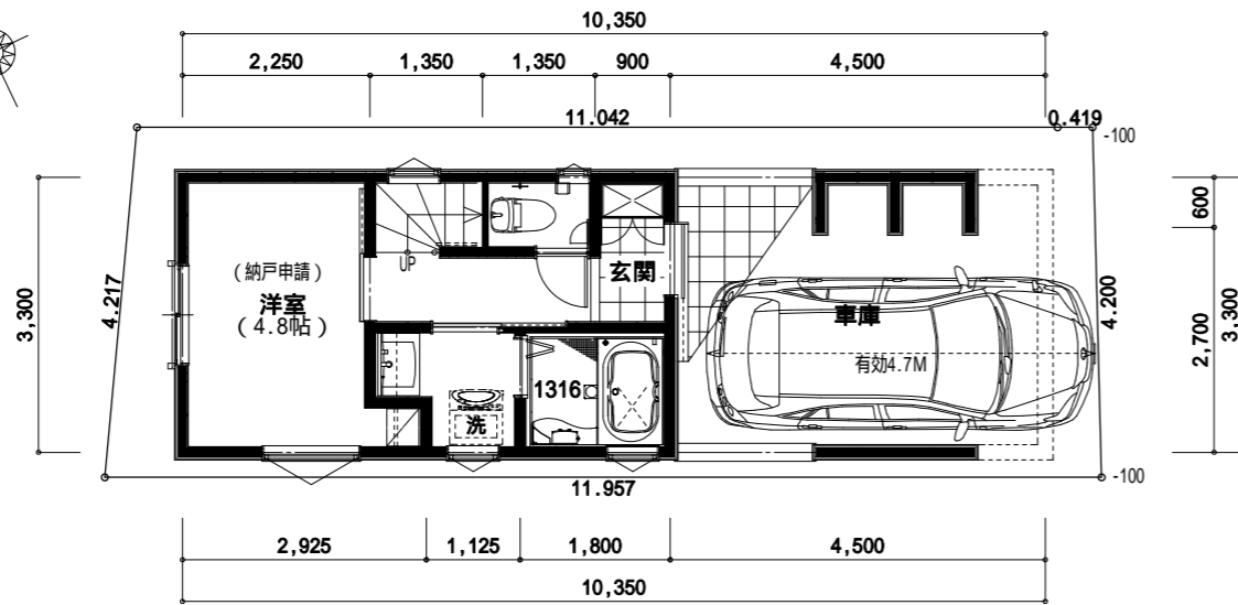
1階 平面図
