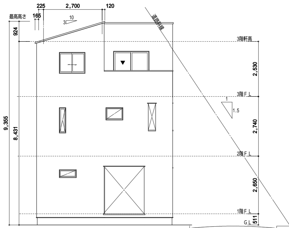
南側立面図
