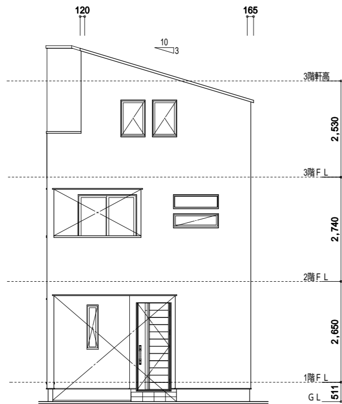
東側立面図
