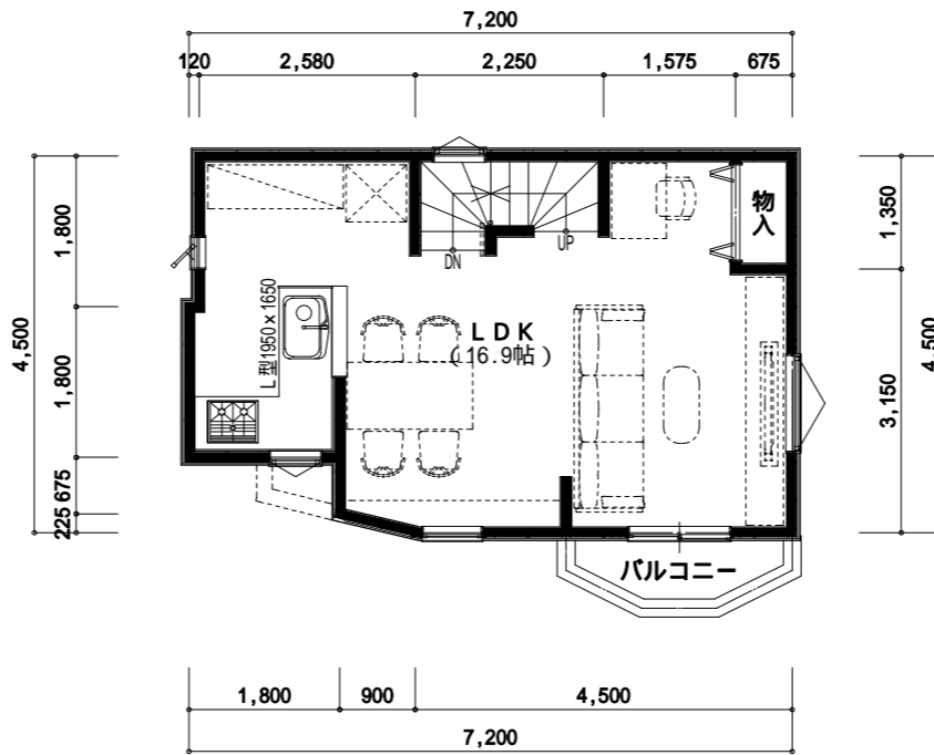
2階 平面図
