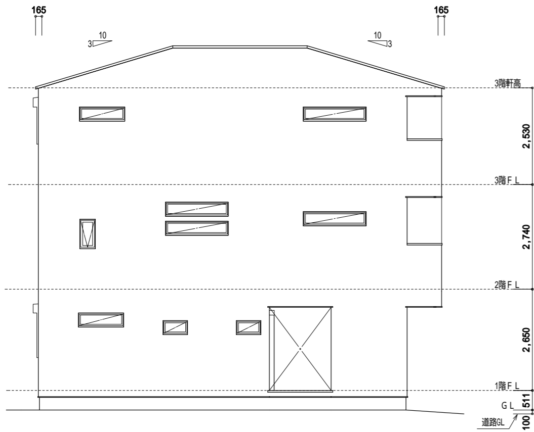
南側 立面図
