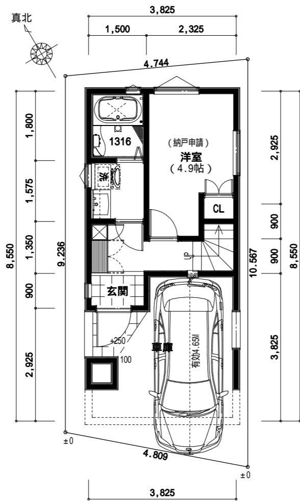
1階 平面図
