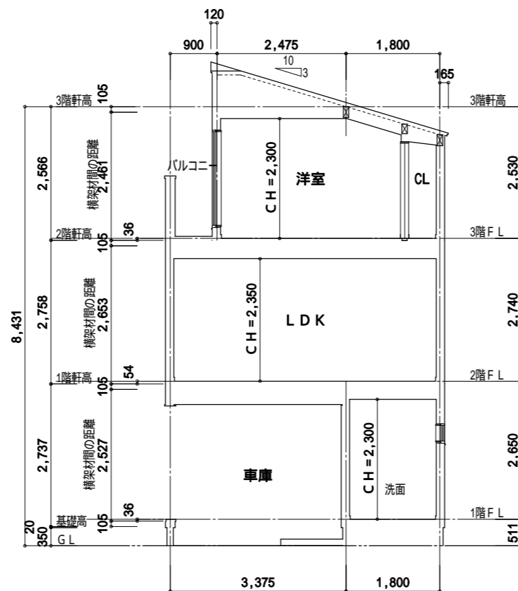
1面断面図
