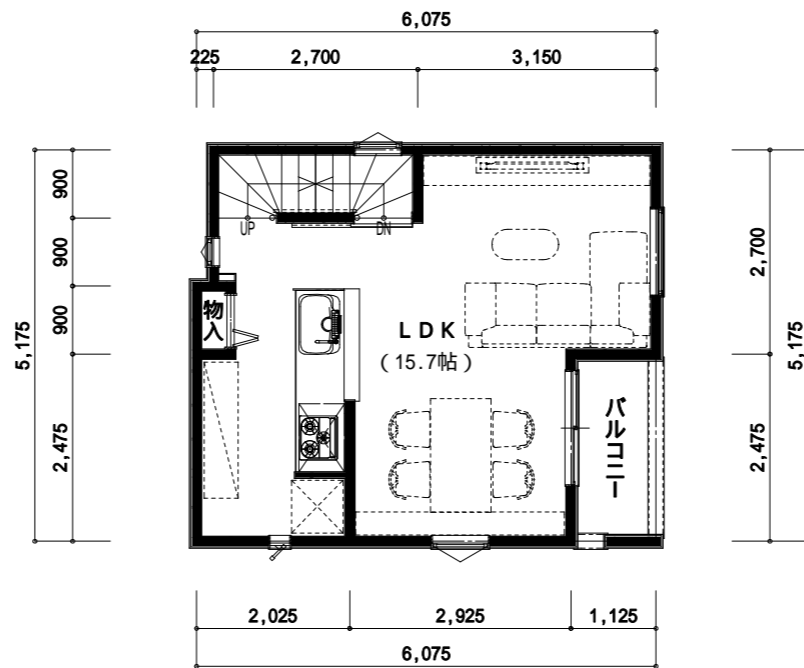
2階 平面図
