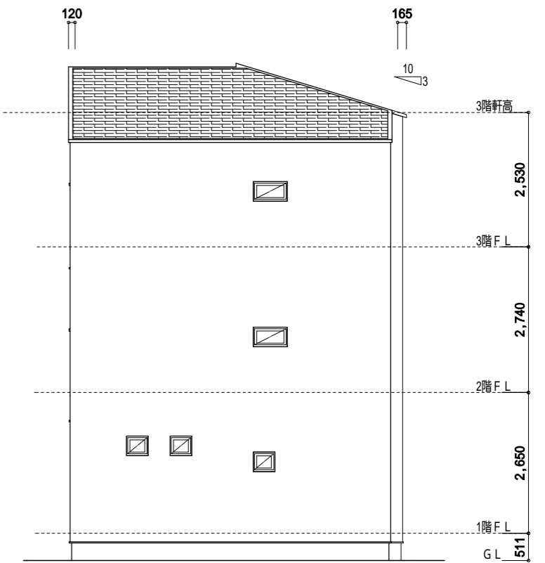
北側立面図
