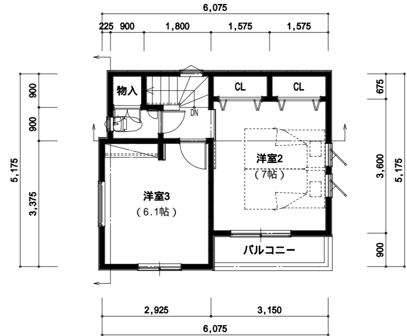
3階 平面図
