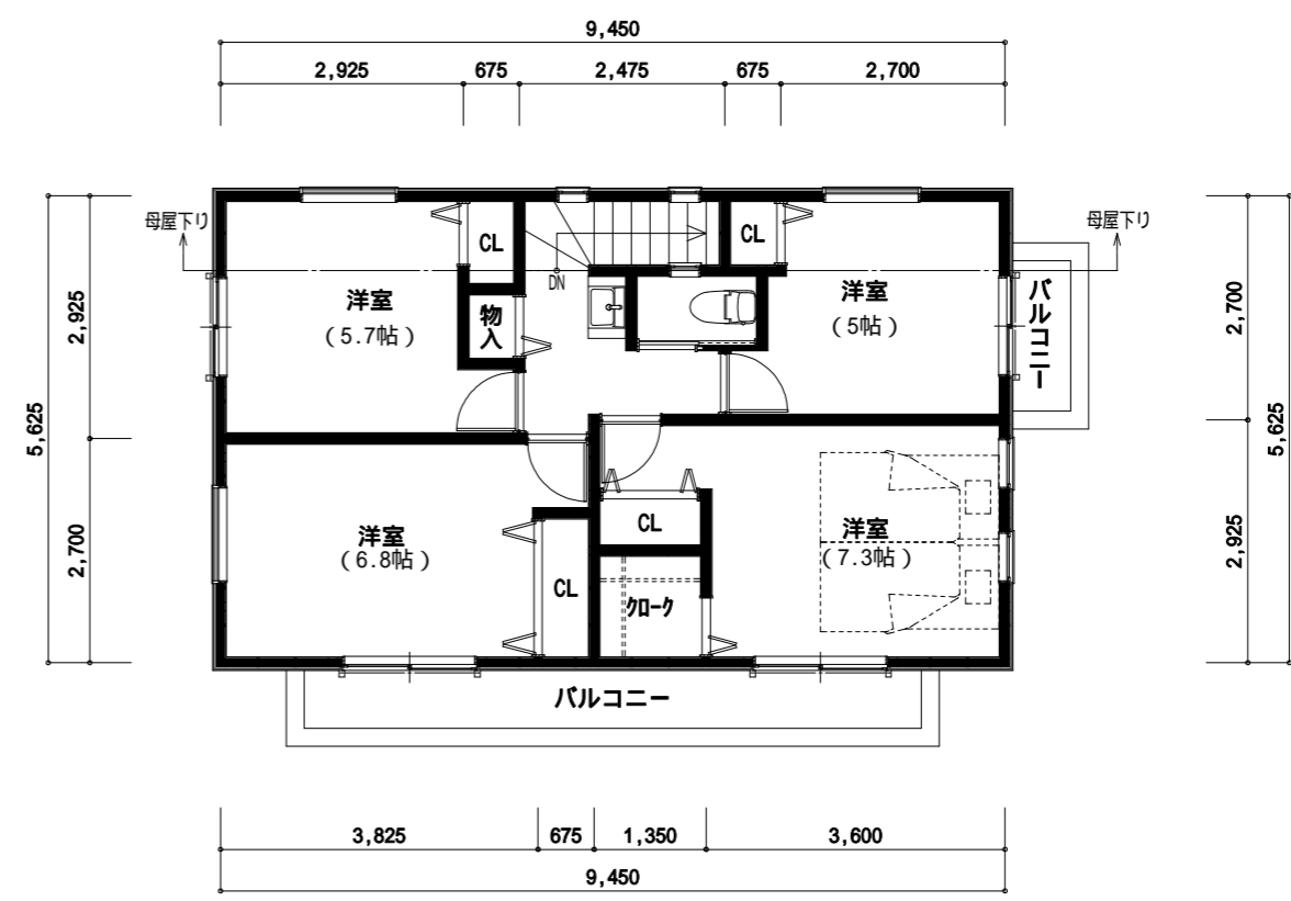
2階 平面図
