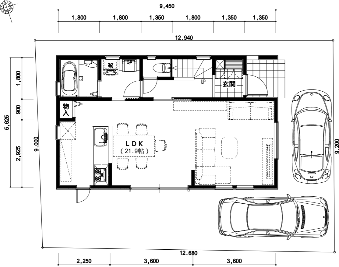
1階 平面図
