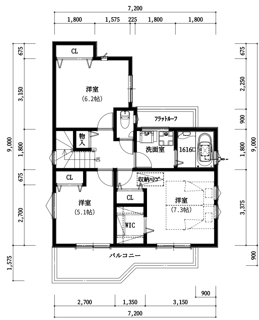
2階 平面図
