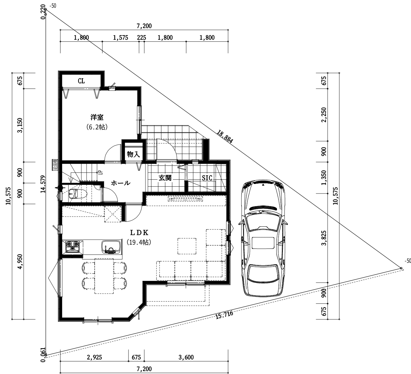
1階 平面図
