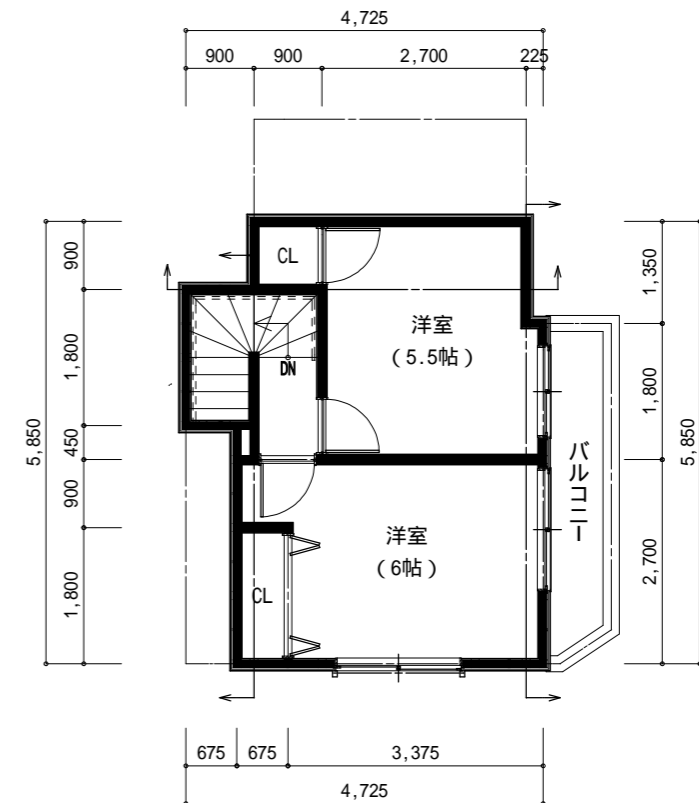
3階 平面図
