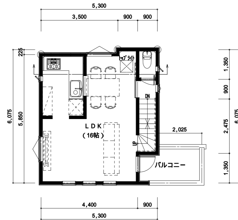
2階 平面図
