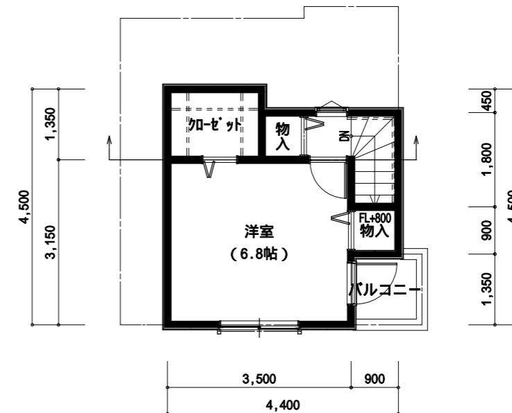
3階 平面図
