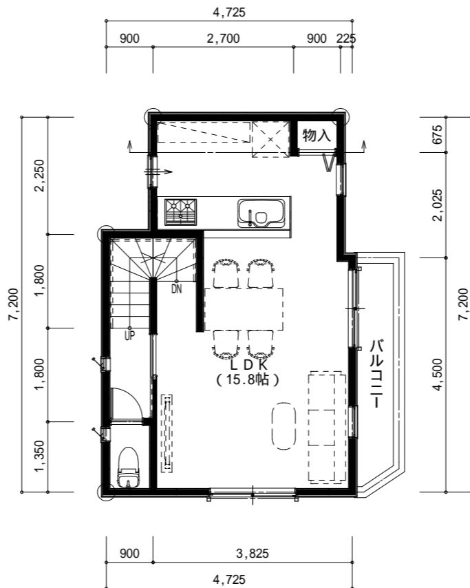
2階 平面図
