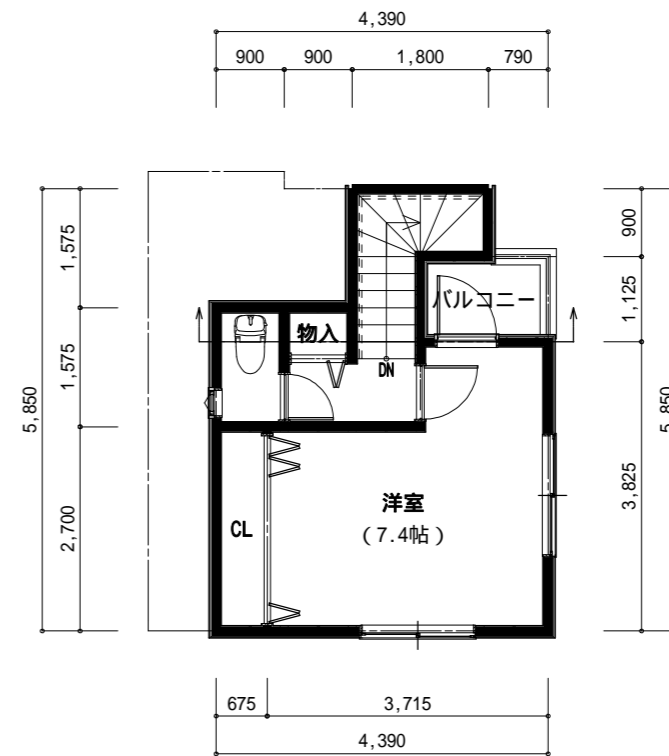
3階 平面図
