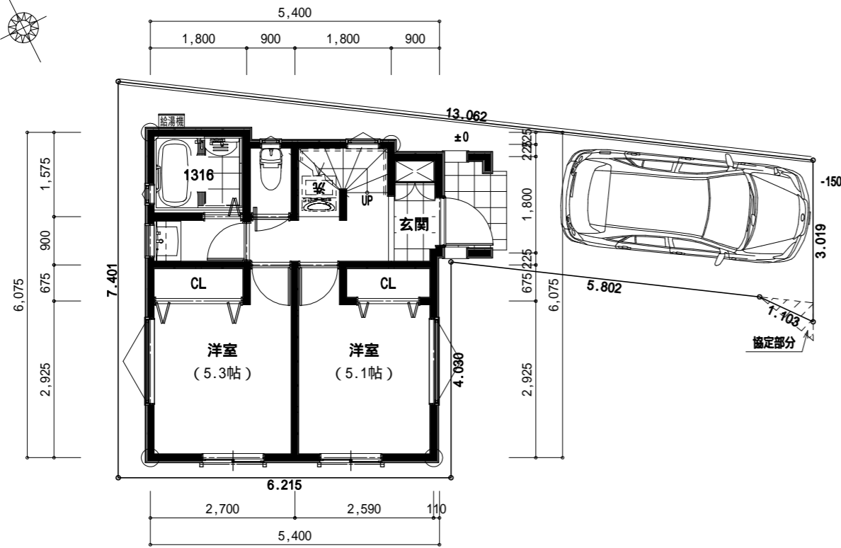
1階 平面図
