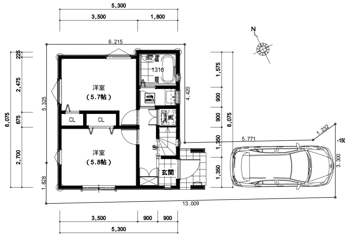
1階 平面図
