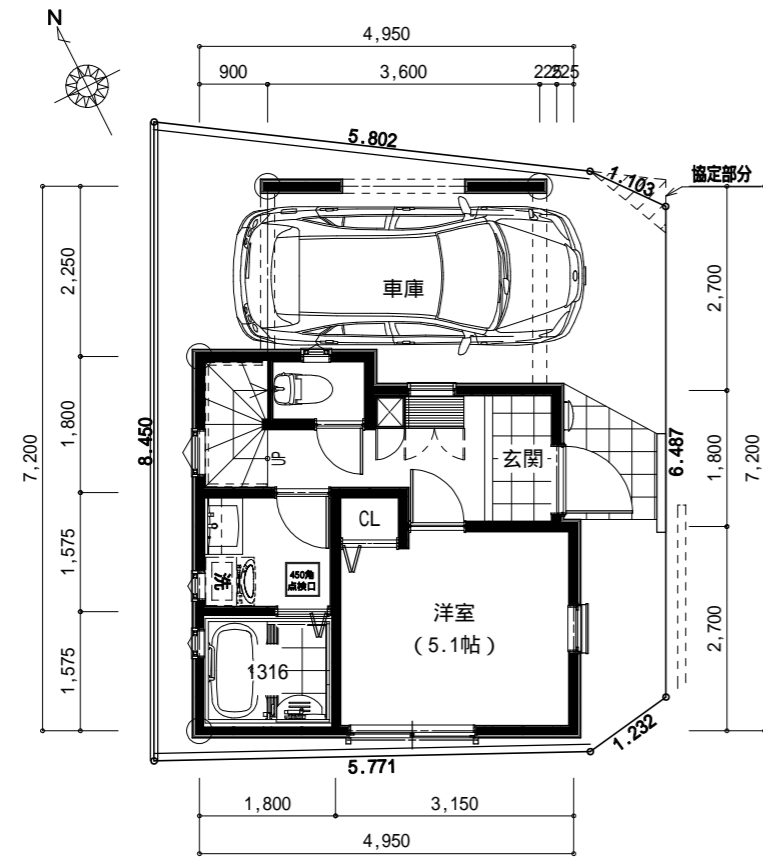
1階 平面図
