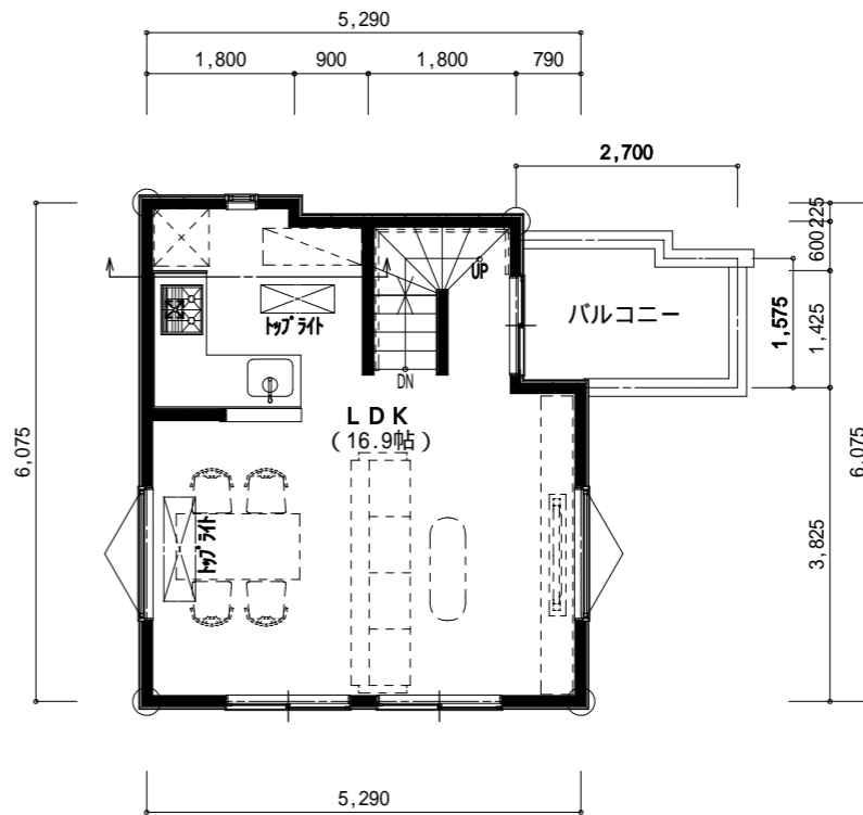
2階 平面図
