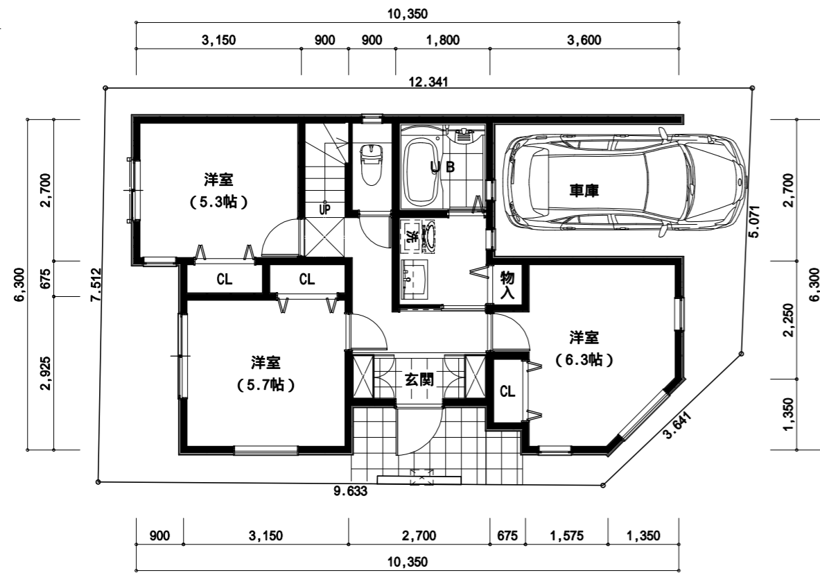
1階 平面図
