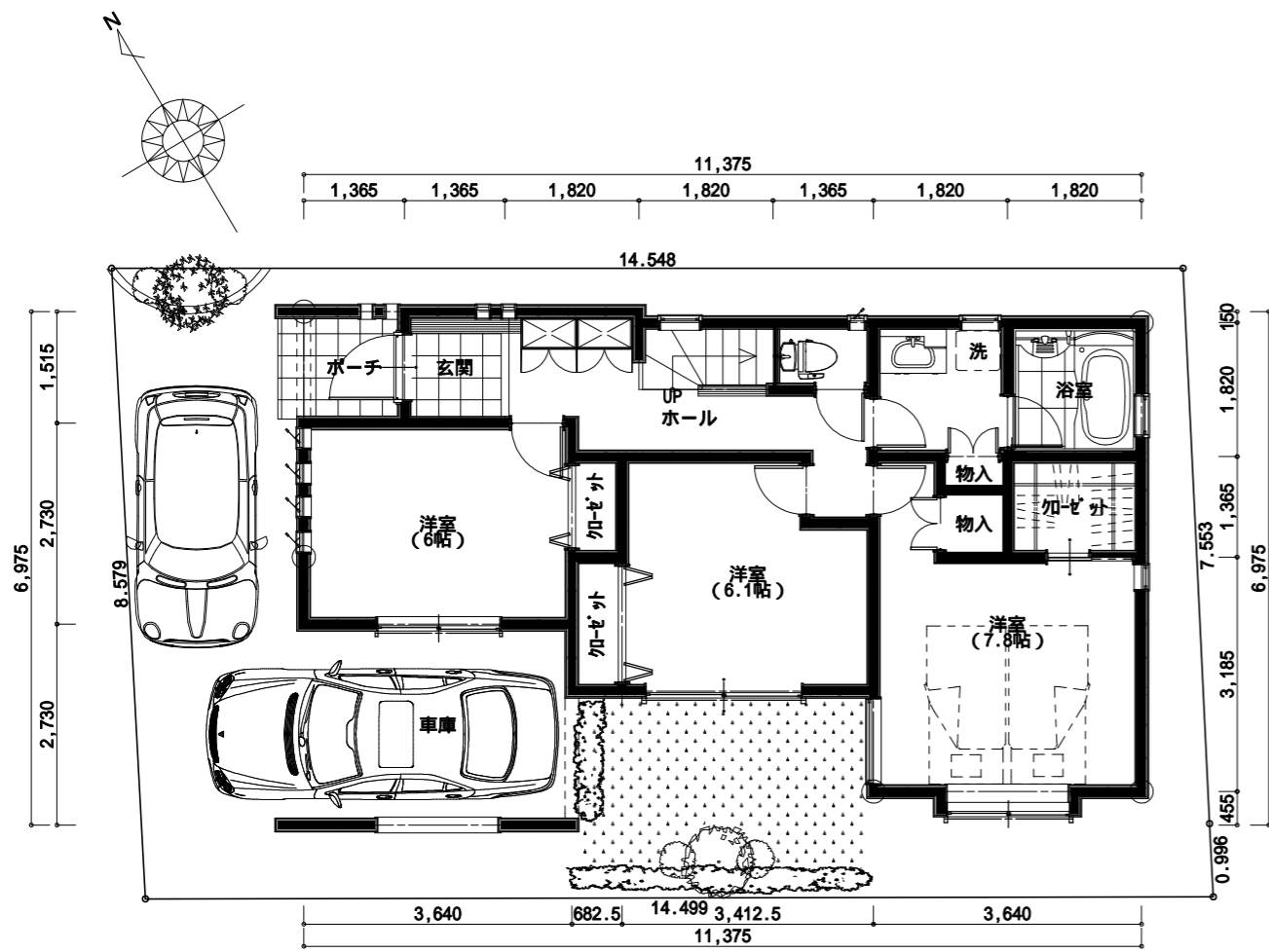
1階 平面図
