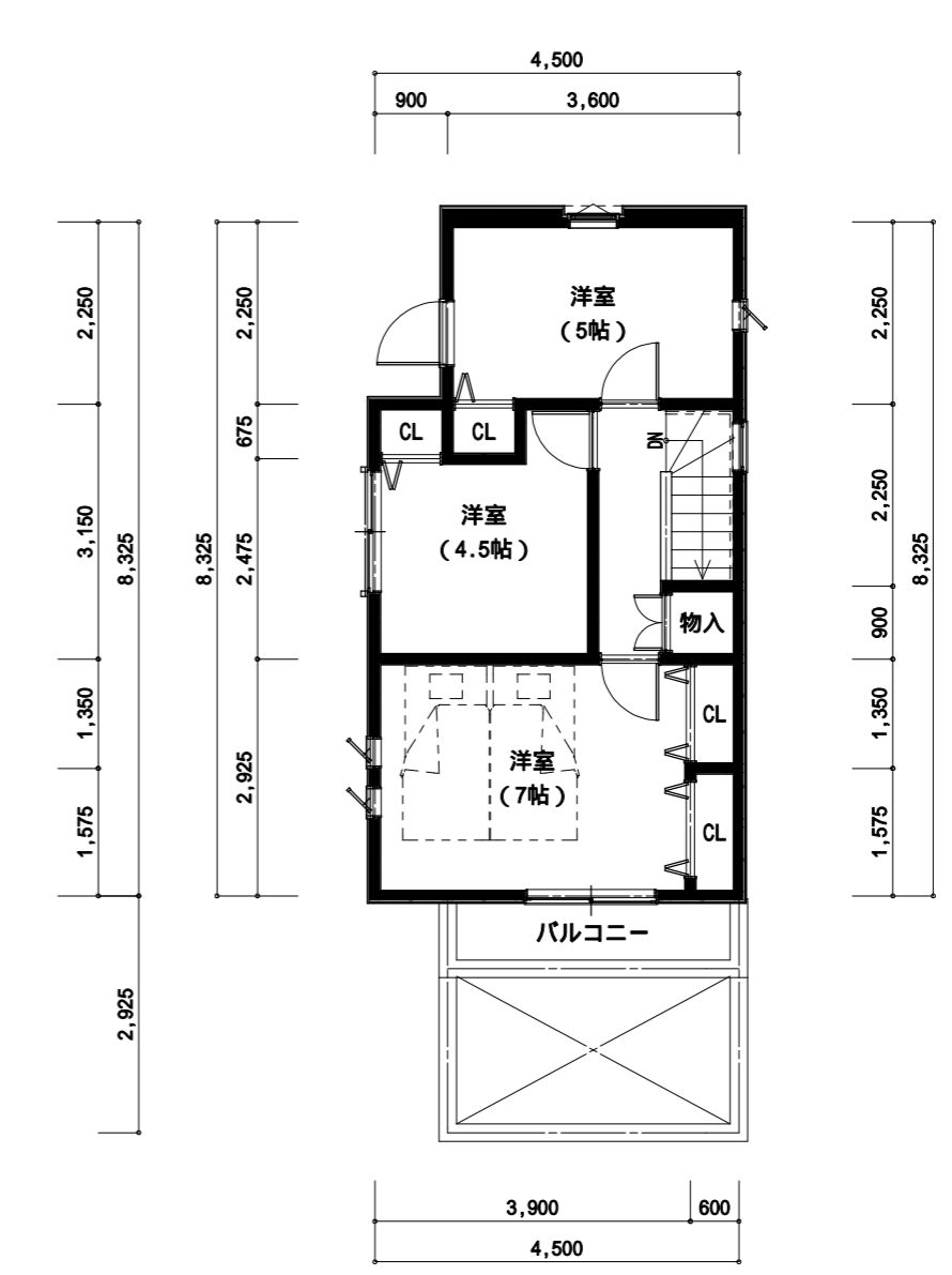
3階 平面図
