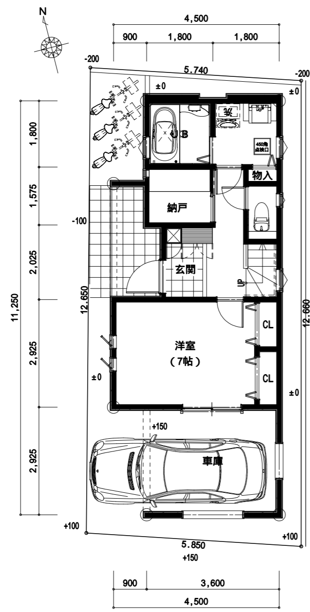
1階 平面図
