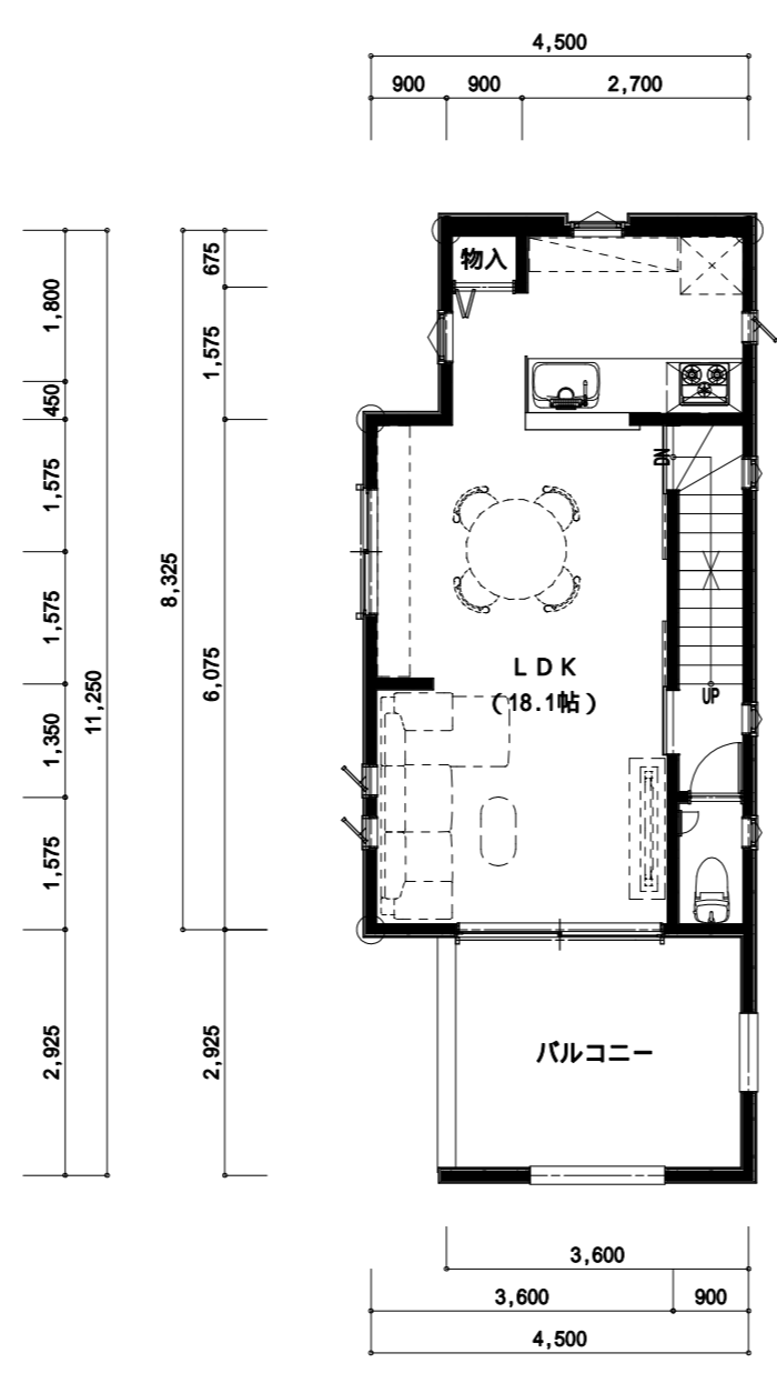
2階 平面図
