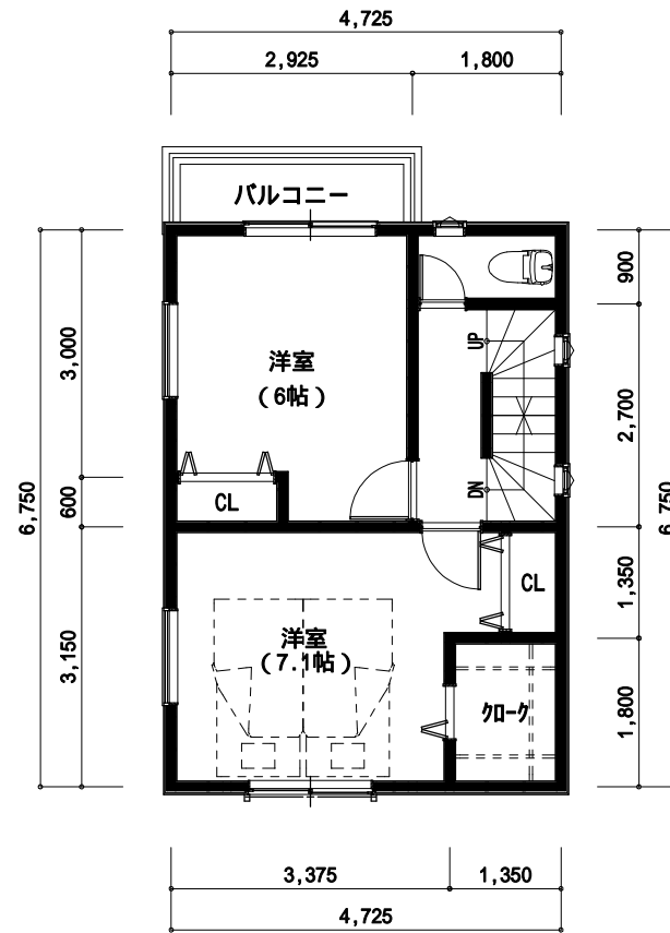
3階 平面図
