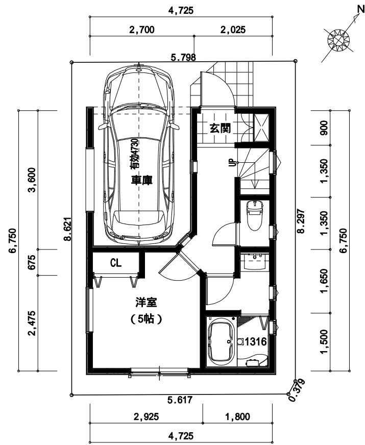
1階 平面図
