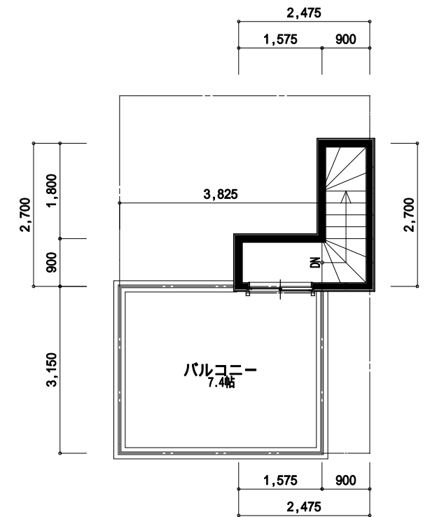
PH1階 平面図
