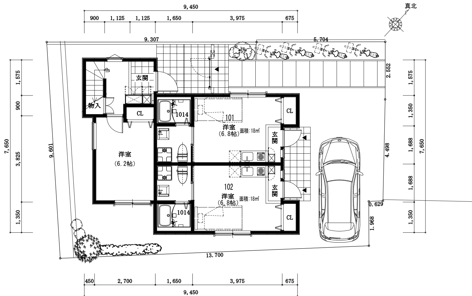
1階 平面図
