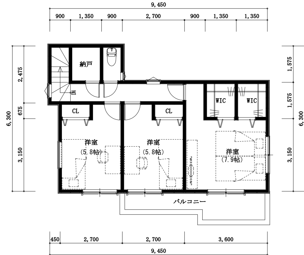
3階 平面図
