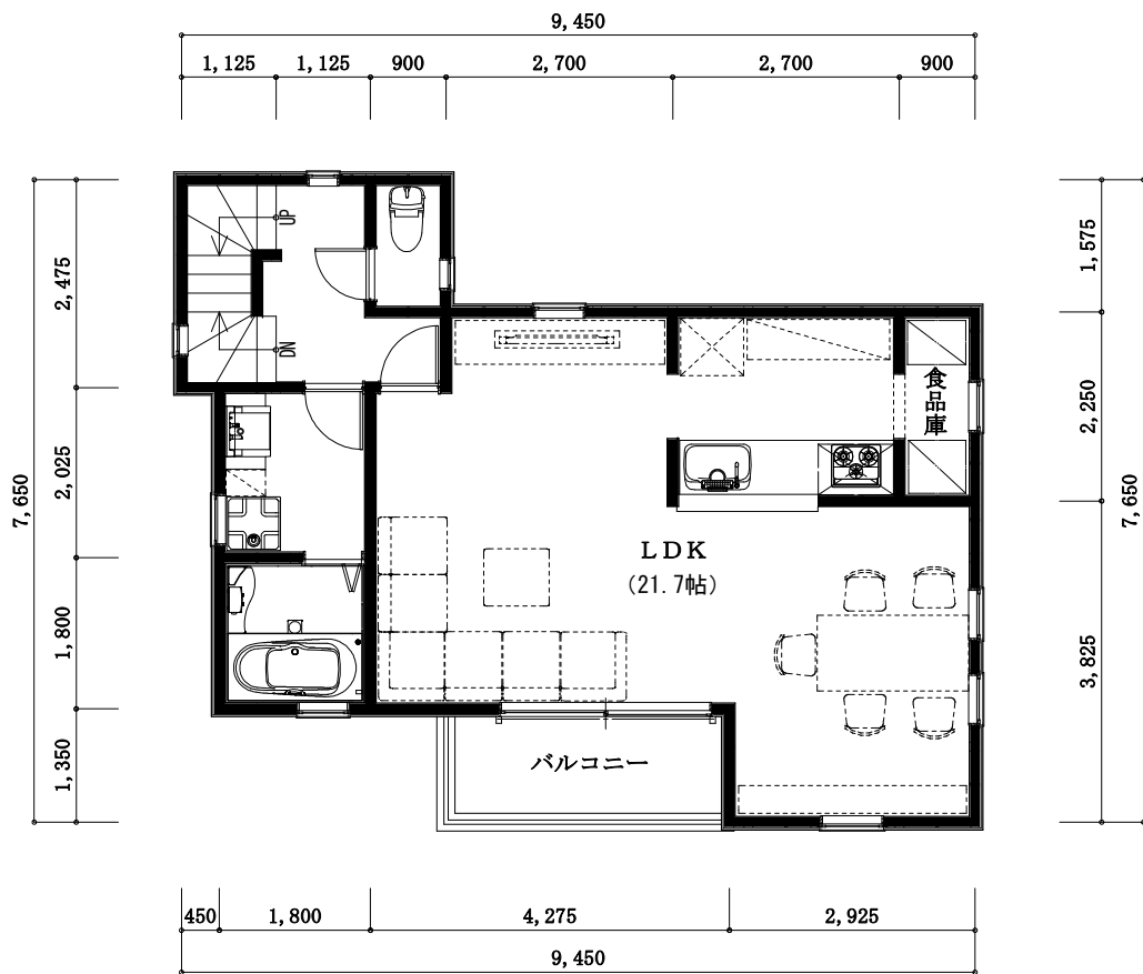
2階 平面図
