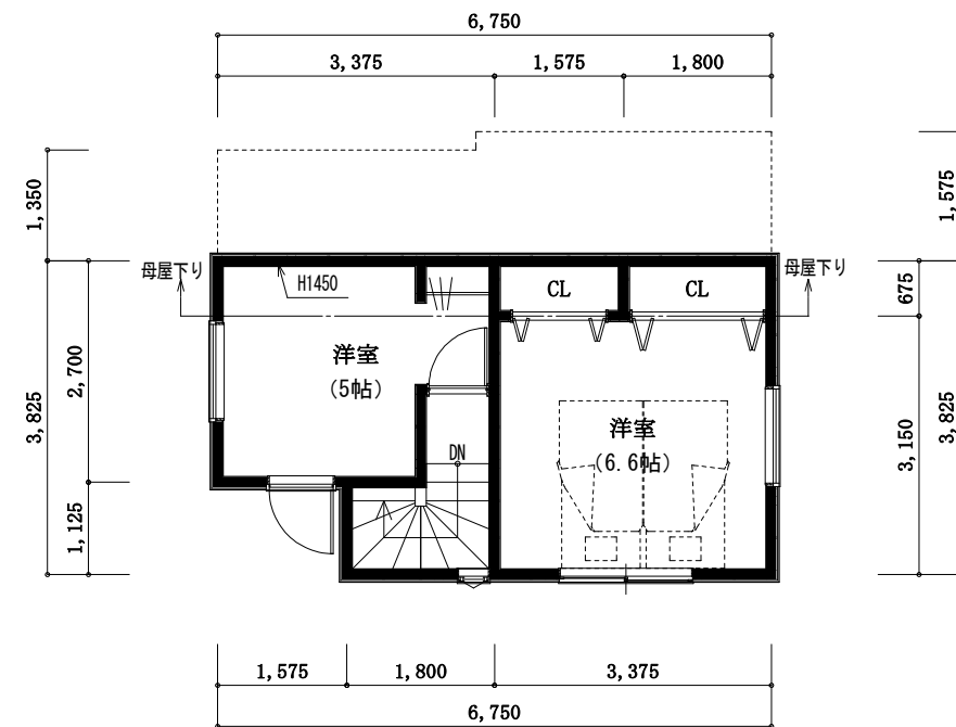
3階 平面図
