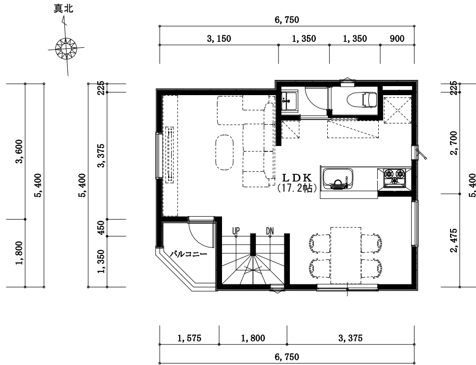
2階 平面図
