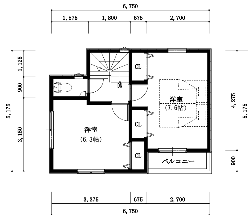
3階 平面図
